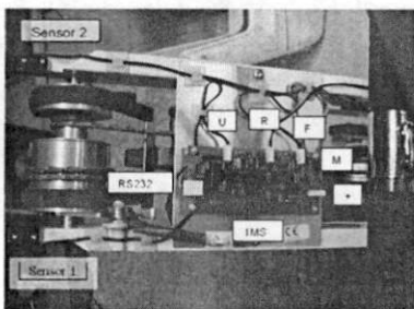
Fig: Conexiones en la placa de circuito
