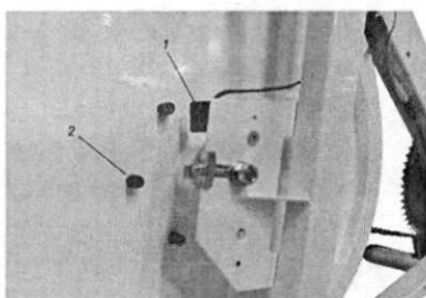
Fig: Sensor e imanes en el volante de inercia
