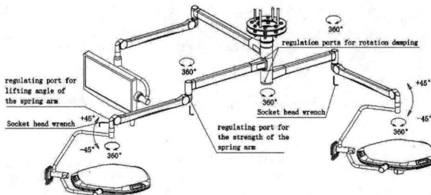
Figura 4-7 Serie OL96 Diagrama de ajuste de la lámpara quirúrgica LED sin sombra
